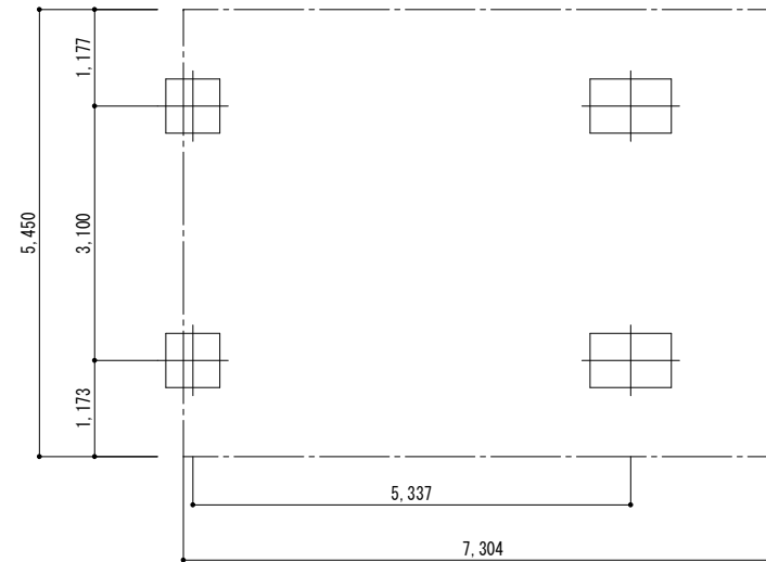
■ 基礎配置図
